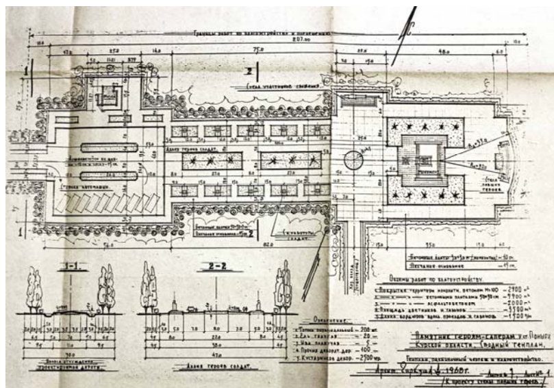
Проект реконструкции и благоустройства территории у памятника Героям-саперам. Автор Д.И. Гаркуша. 1968 г.
